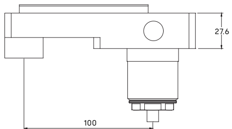
Top View Vista de Cima
