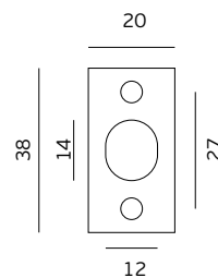
Chapa de fixação ao chão / Floor fixing plate / Placa de fijación al suelo
