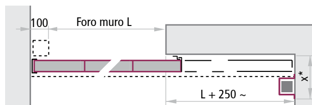
Versione contrappeso disassato rinvitato x=330 (REI 120), x=390 (REI 180)
