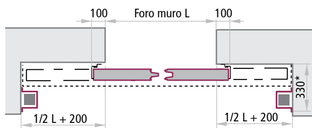
Versione 2 ante contrappesi disassati REI 120
