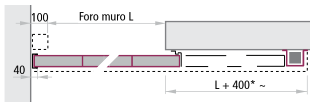
Versione contrappeso rinvitato con battuta normale
