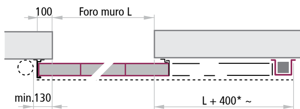
Versione contrappeso rinvitato con battuta speciale
